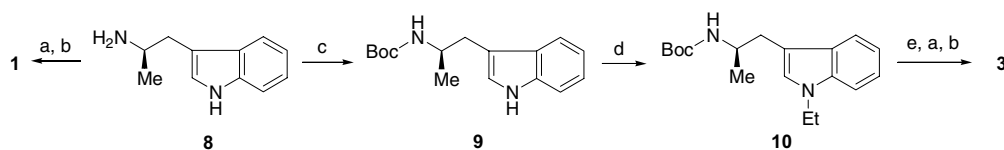
Scheme 2. Reagents: (a) 4 , KI, i -Pr 2 NEt, MeCN; (b) 4M HCl–EtOAc, EtOH; (c) (Boc) 2 O, \text{CHCl}_3 ; (d) EtI, NaH, THF; (e) 4M HCl–EtOAc.
