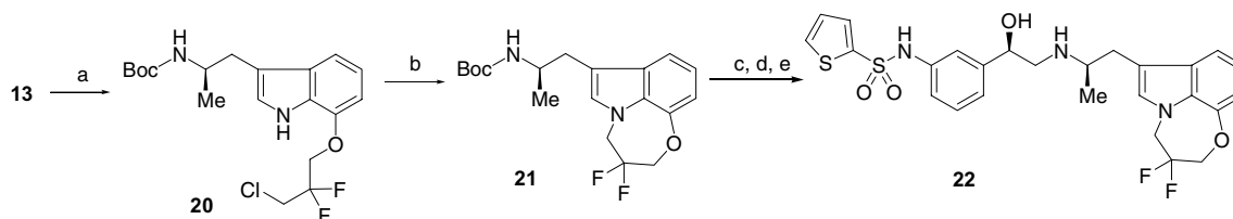
Scheme 5. Reagents: (a) HOCH 2 CF 2 CH 2 Cl, Bu 3 P=CHCN, toluene; (b) KOH, DMSO; (c) 4M HCl-EtOAc; (d) 4 , KI, i -Pr 2 NEt, MeCN; (e) 4M HCl-EtOAc, EtOH.
