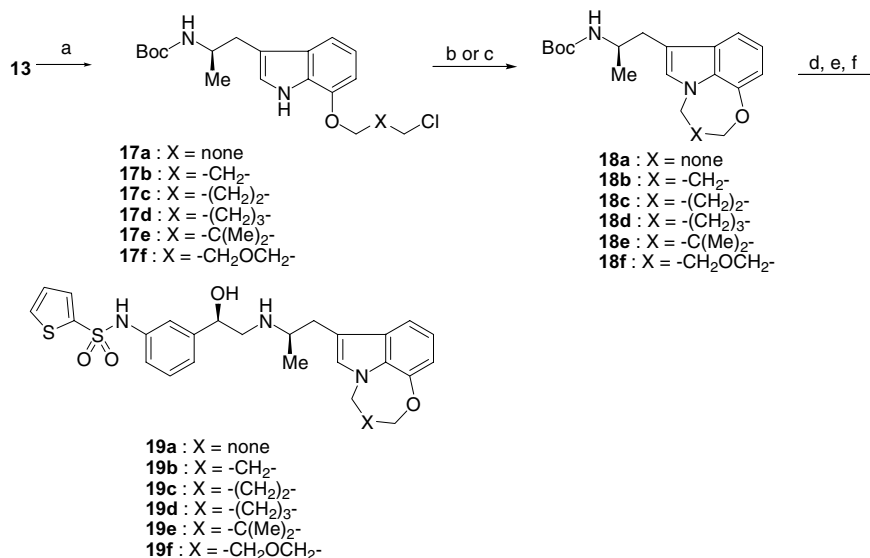
Scheme 4. Reagents: (a) HOCH 2 -X-CH 2 Cl, DEAD, Ph 3 P, THF; (b) NaH, DMF; (c) KOH, DMSO; (d) 4M HCl-EtOAc; (e) 4 , KI, i -Pr 2 NEt, MeCN; (f) 4M HCl-EtOAc, EtOH.
